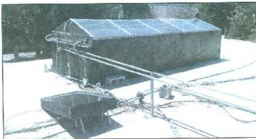
Figura 4.1 Destilador Solar de Alto Rendimiento instalado en el ITL.
