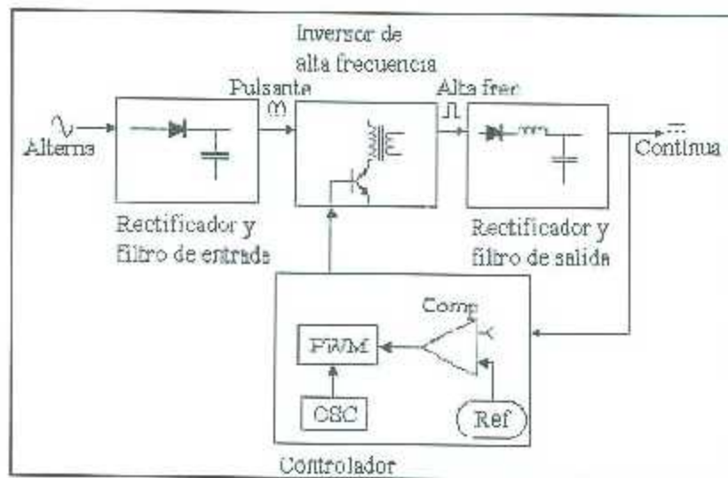
Figura 2.11. Diagrama a bloques de fuente de alimentación conmutada.
