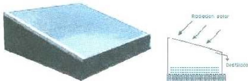
Figura 2.4. Destilador solar de una vertiente o tipo Batea. Efecto Simple
