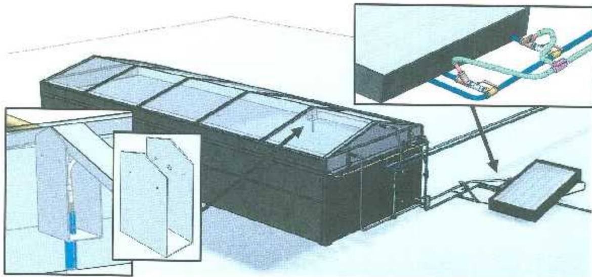
Figura 3.8. Diseño en SolidWorks de la base para sensor ultrasónico de nivel de agua en la charola (Izquierda) y la forma de montaje de los sensores de temperatura de la entrada y la salida de agua del colector solar.
