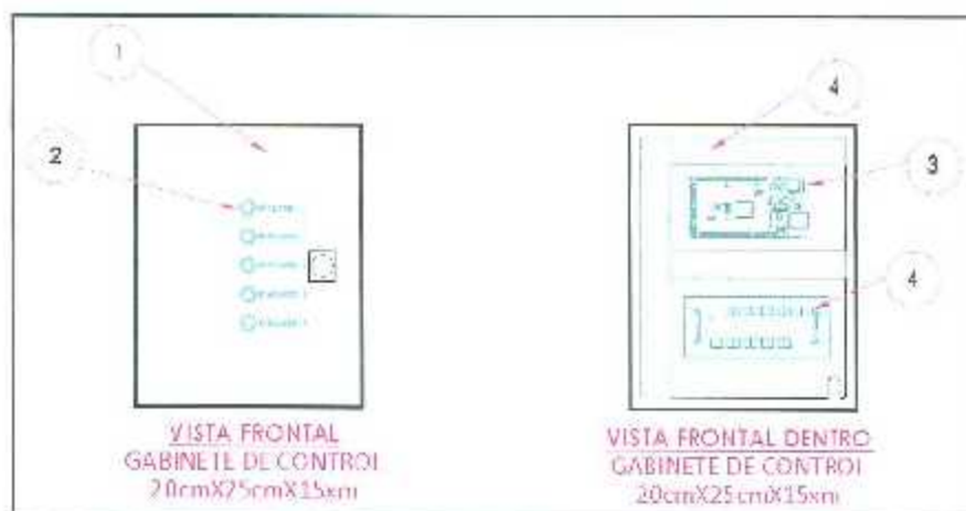
Figura 3.49. Layuot de gabinetes de control del sistema.
