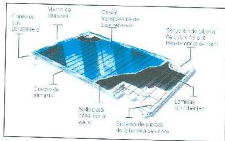
Figura 2.9. Esquema de un colector solar plano.
