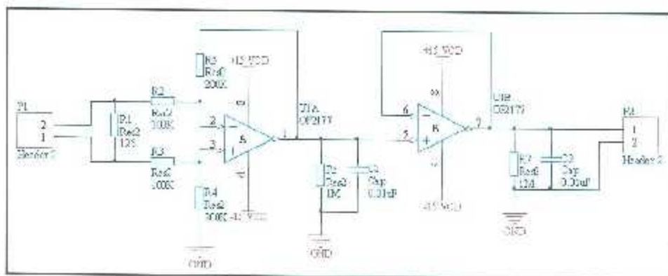
Figura 3.41 Diagrama esquemático del circuito de conversión de señal 4-20 mA a señal analógica 0-5V.
