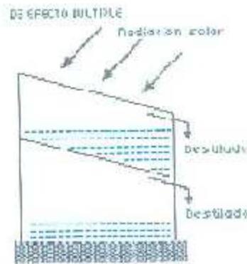
Figura 2.5. Destilador Solar tipo Batea Multifecto.
