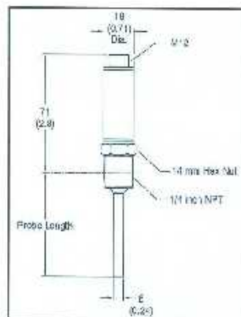
Figura 3.29. Dimensiones aproximadas del interruptor de temperatura sin pantalla 837E [mm (in)].
