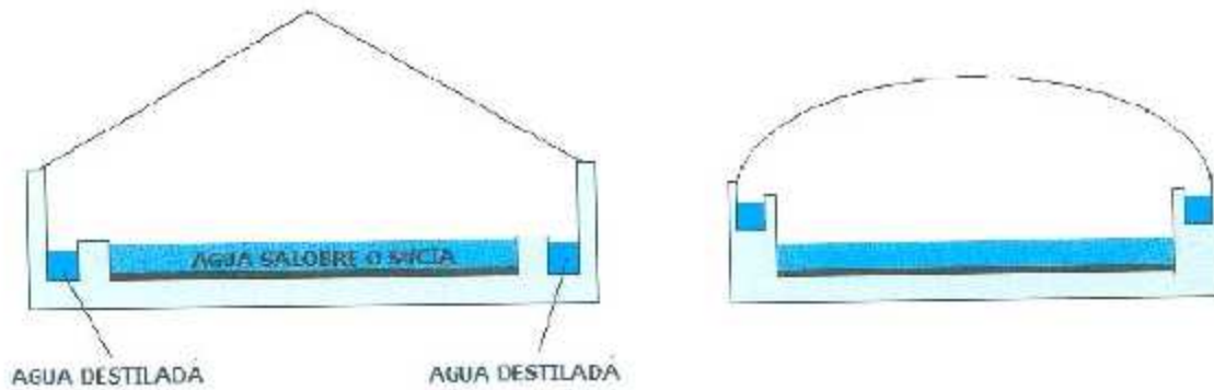
Figura 3.3. Destilador de dos vertientes la cubierta puede ser de dos aguas o de bóveda.
