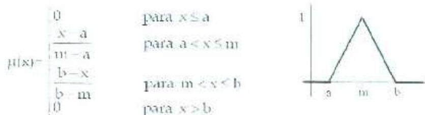
Figura 2.14. Función de transferencia para un conjunto difuso triangular.
