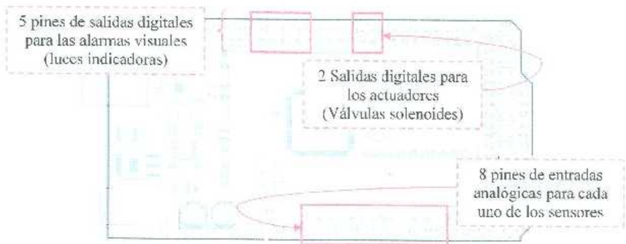
Figura 3.38. Configuración de los pines de la placa Arduino MEGA 2560.
