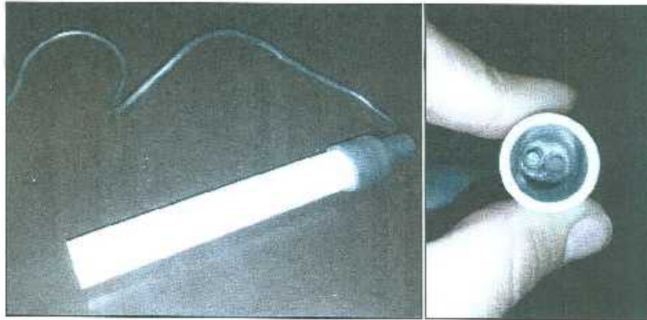
Figura 3.34. Base con electrodos con recubrimiento reutilizada en el sensor de conductividad eléctrica desarrollado para la aplicación.
