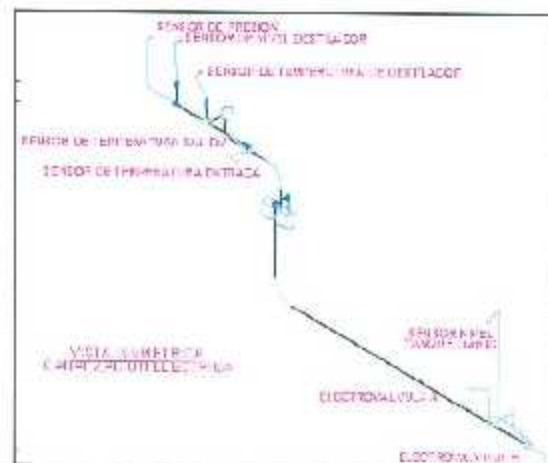
Figura 3.45. Cableado y canalización del sistema de instrumentación.
