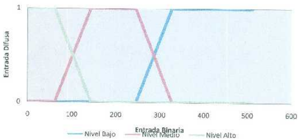
Figura 3.53. Gráfica de la función de pertenencia de la variable nivel de agua en charola
