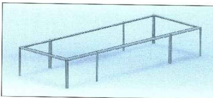
Figura 3.4. Diseño en SolidWorks de la estructura que soportará la charola del destilador solar.
