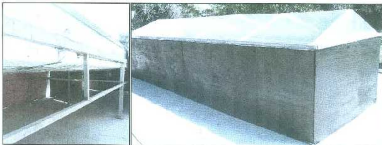
Figura 3.23. A (Izquierda): Instalación aislante térmico debajo de la charola. B (Derecha): Cubierta de madera para cubrir el sistema de las corrientes de aire.
