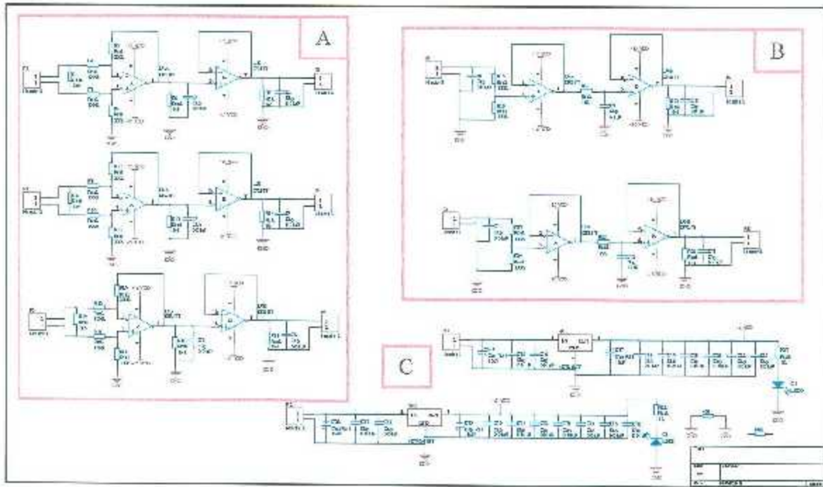
Figura 3.40. Diagrama esquemático de la tarjeta de acondicionamiento de señales. A) Conversión 4-20 mA a 0-5V. B) Conversión 0-10V a 0-5V. C) Alimentación de la tarjeta.
