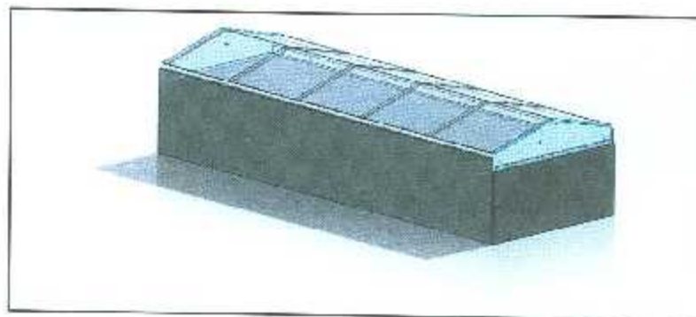
Figura 3.5. Modelo 3D de la distribución de los soportes para la cubierta de vidrio del destilador solar.
