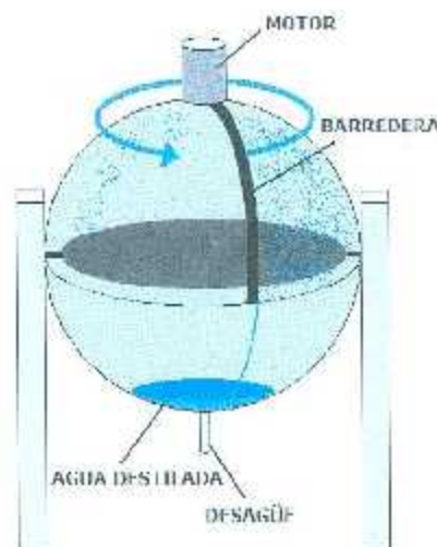
Figura 2.8. Destilador solar tipo Barredora.
