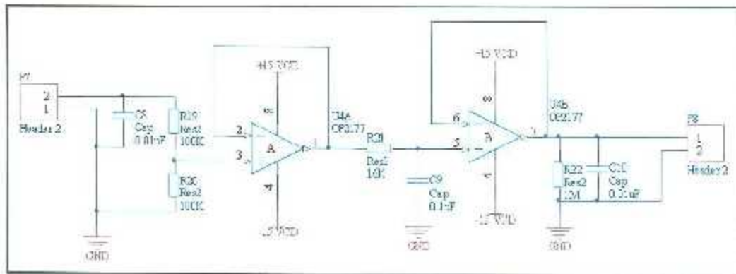
Figura 3.42 Diagrama esquemático del circuito de conversión de señal analógica 0 a 10V a 0-5V.
