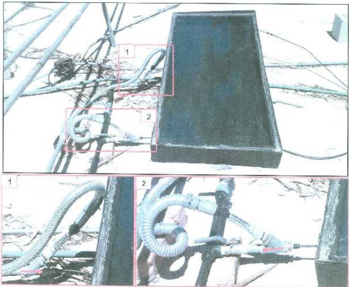
Figura 3.30. Sensores de temperatura de entrada (1) y temperatura salida (2) del colector solar plano.
