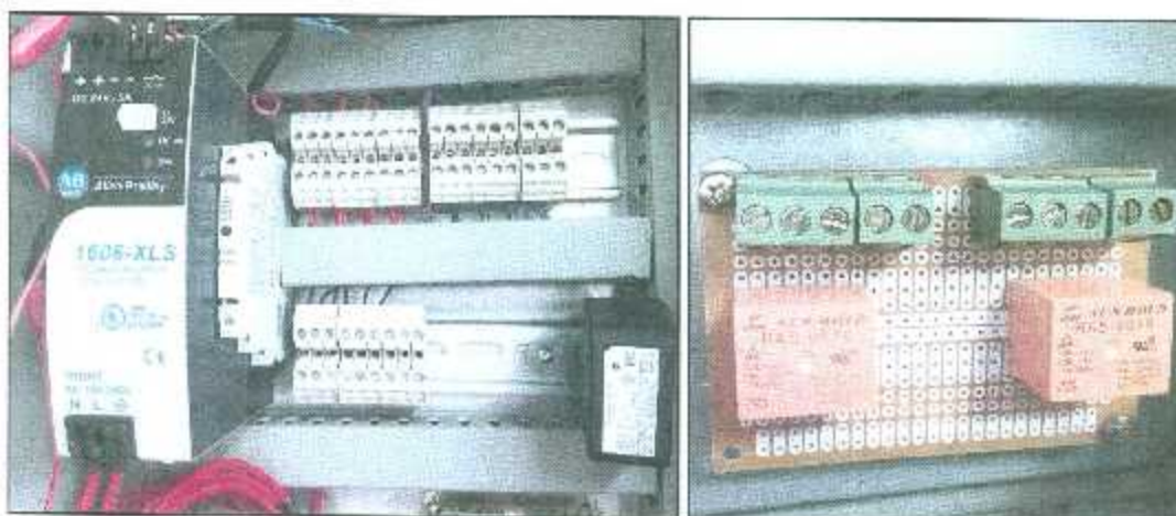
Figura 3.50. Gabinetes de control del sistema de instrumentación en etapa de ensamble.
