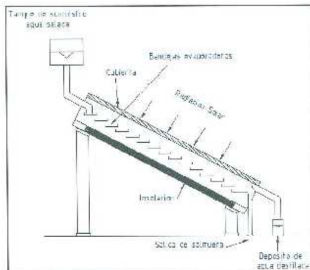
Figura 2. 7. Destilador solar tipo cascada
