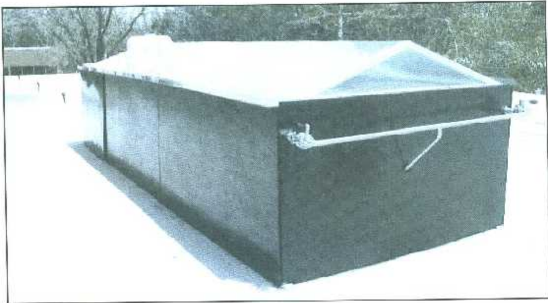
Figura 2.2. Destilador solar instalado en el Tecnológico de la Laguna, año 2008.
