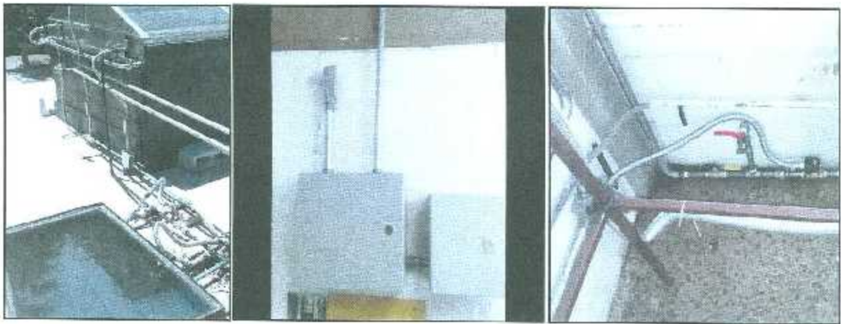
Figura 3.48. Instalación final de tubería y cableado eléctrico.
