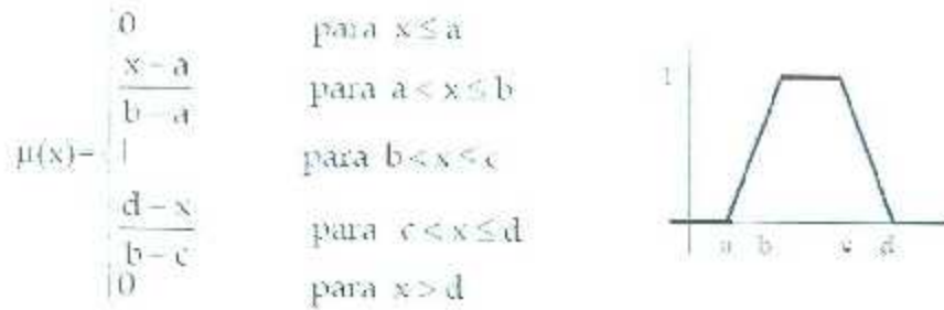
Figura 2.15. Función de transferencia para un conjunto difuso trapezoidal.
