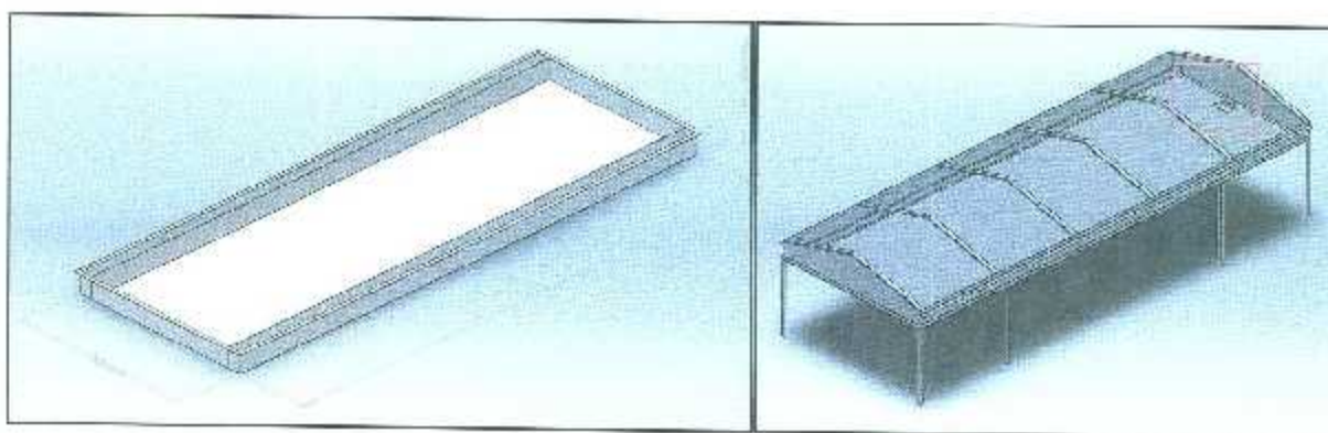
Figura 3.3. Diseño en SolidWorks de la charola del destilador solar de alto rendimiento (a) Dimensiones generales, (b) Diseño que incluye cárcamo para facilitar la purga del sistema.
