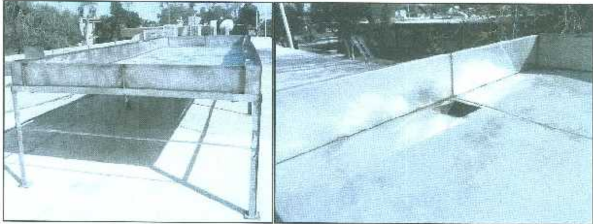
Figura 3.11. Charola y estructura de soporte en etapa de construcción.
