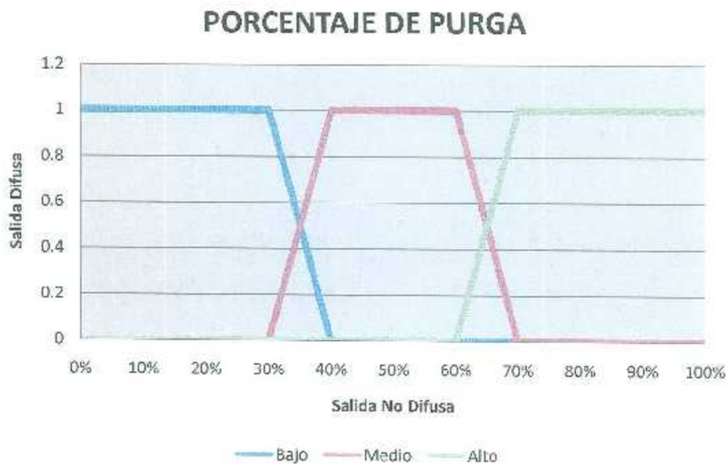
Figura 3.56. Grafica de defusificación de la salida.
