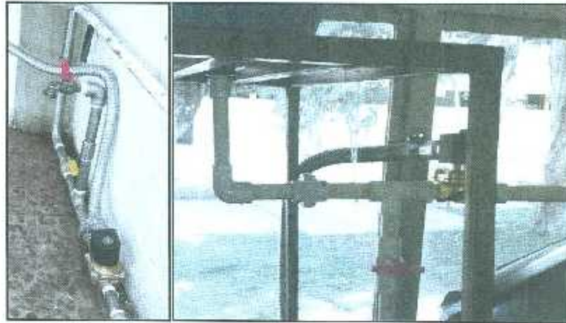
Figura 3.35. A. (Izquierda) Válvula solenoide en línea de purga de charoia. B (Derecha) Válvula solenoide instalada on tubería que une tanque de almacenamiento diario con tanque general.
