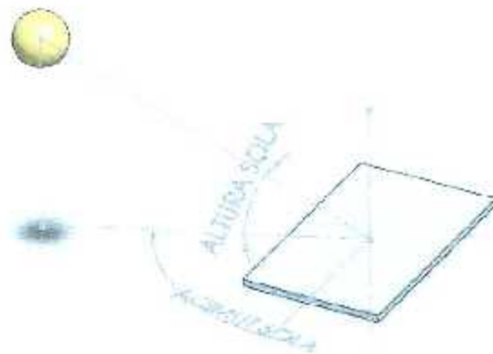
Figura 2.1. Ángulos que definen la posición del sol.
