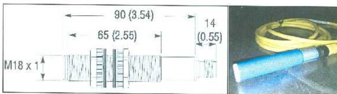
Figura 3.26. Dimensiones del sensor de proximidad ultrasónico 873P.
