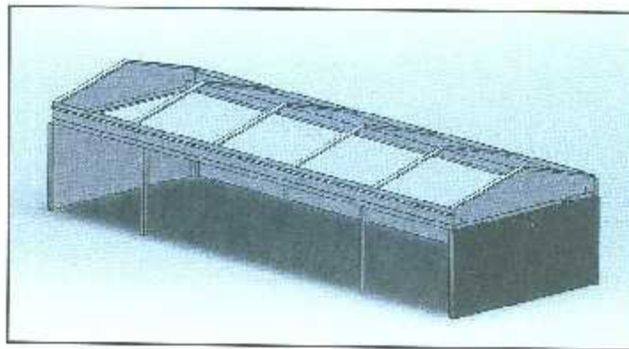
Figura 3.5. Modelo 3D de la distribución de los soportes para la cubierta de vidrio del destilador solar y recubrimiento de madera para evitar corrientes de aire bajo la charola.
