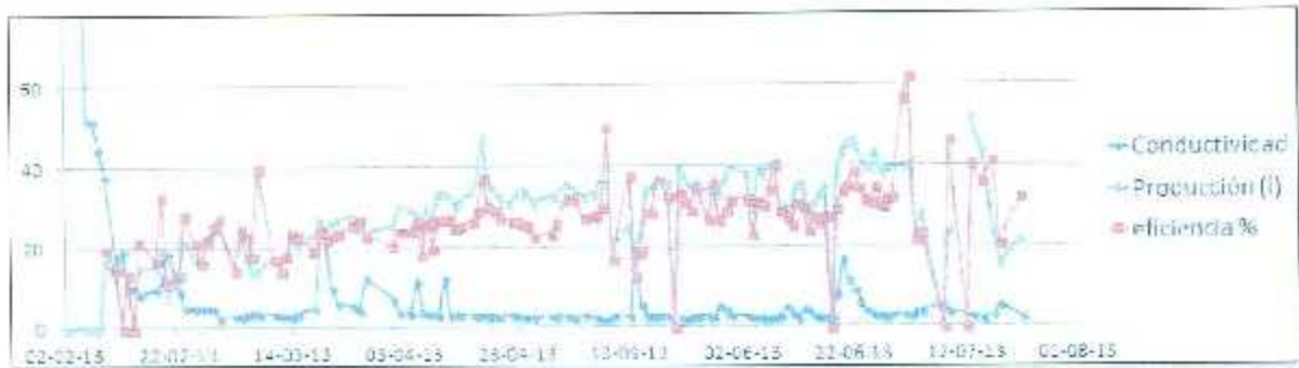
Figura 4.3. Gráfica de conductividad de agua producto, producción de agua destilada y porcentaje de eficiencia.
