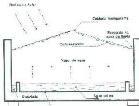
Figura 2.6. Destilador de dos vertientes la cubierta puede tener forma de dos aguas o de bóveda.
