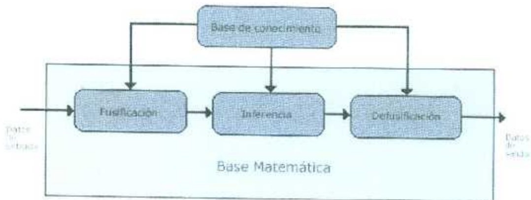
Figura 2.16. La estructura de un controlador difuso.
