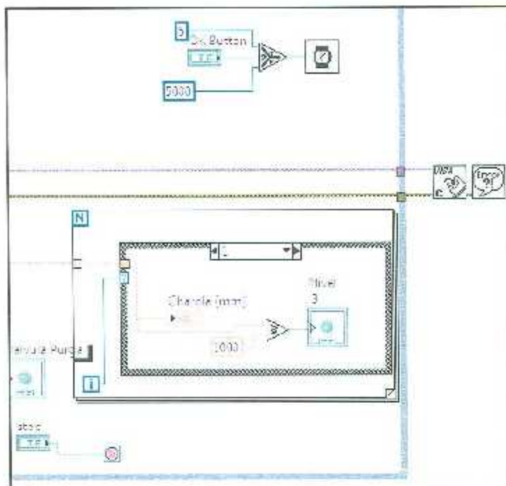
Figura 3.62. Secuencia de inicio para la recepción de los datos desde Arduino.
